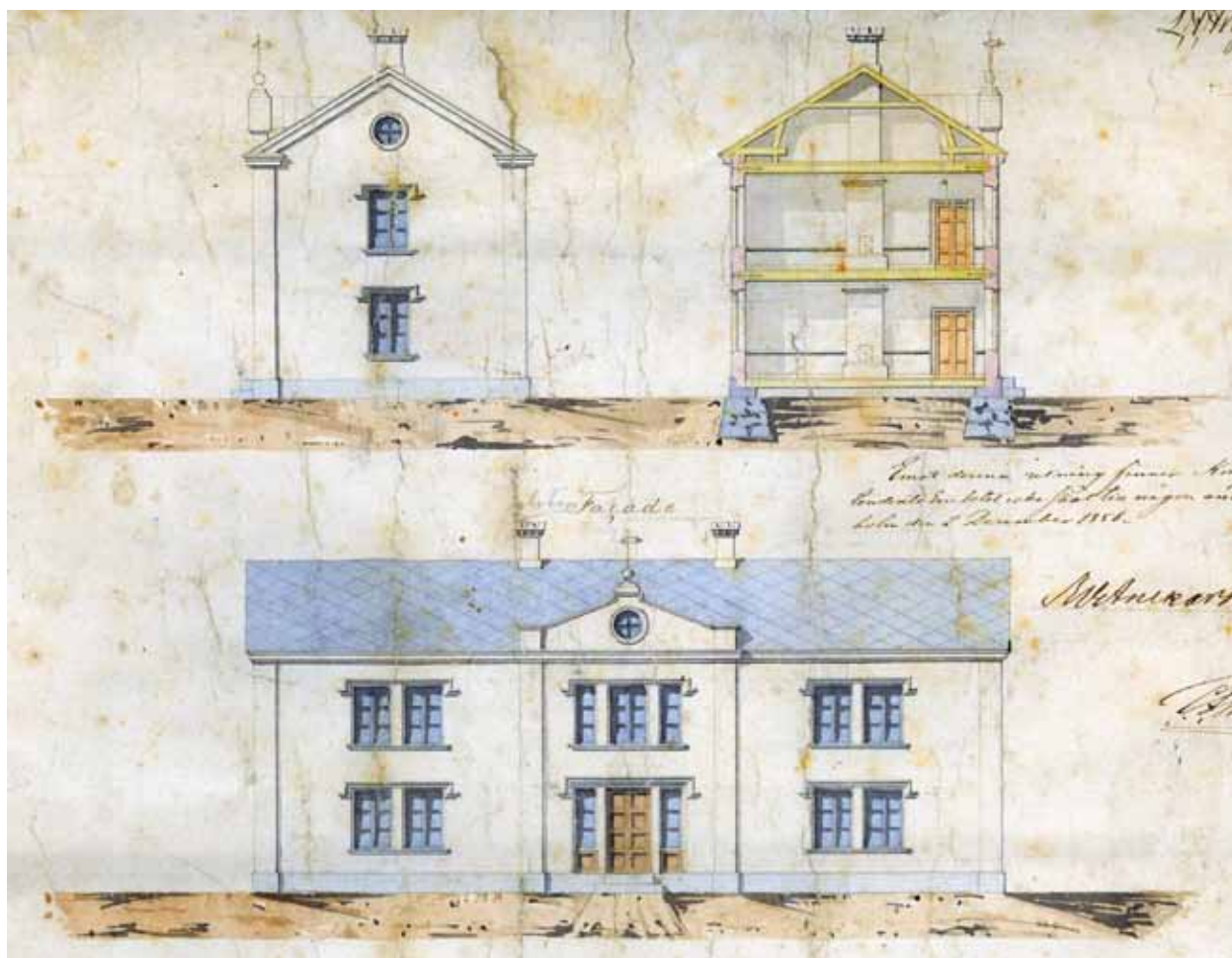
Ritning från 1856 till lasaretsbyggnaden Hvilan vid Loka brunn. Här fanns två badrum »där den bemedlade allmogen helst badar, då priset där är billigare«. Ur Loka brunns arkiv.
